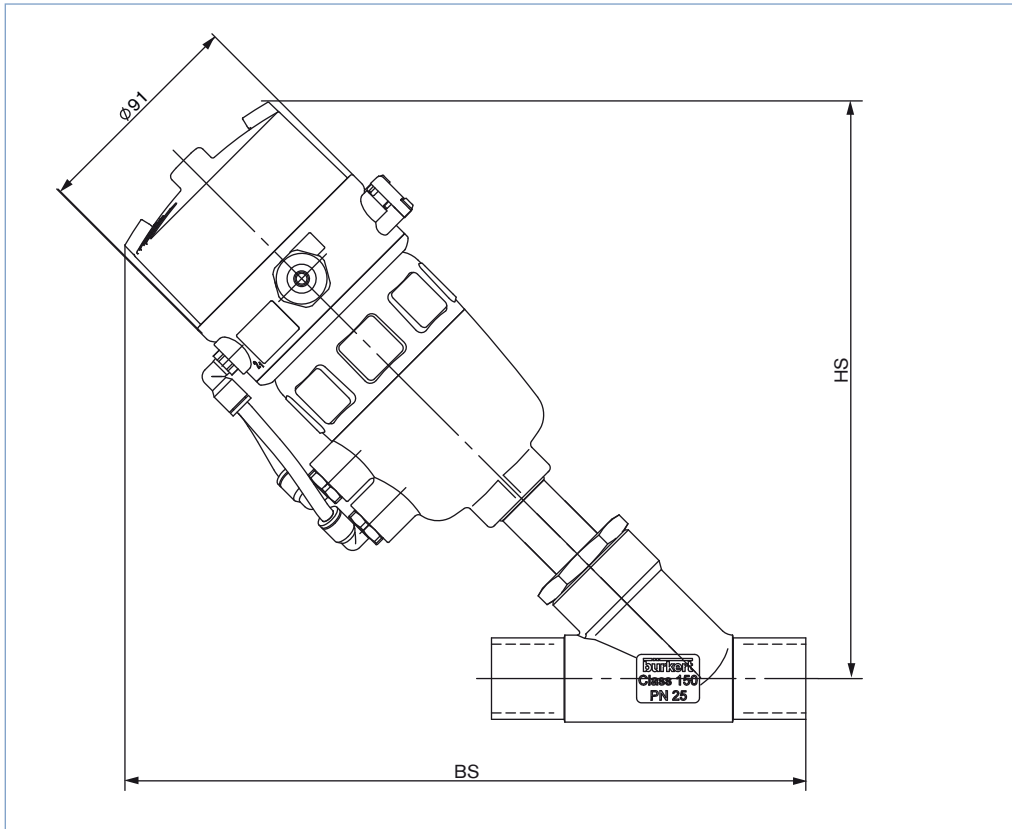
Acc. to EN ISO 1127/ISO 4200, DIN 11850 S2 [mm]
